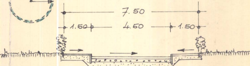
STRASSENPROFIL M. 1:100
